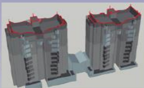
Diseño apantallamiento, edificio Pradera
